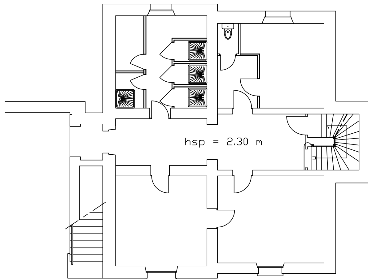
sous sol
