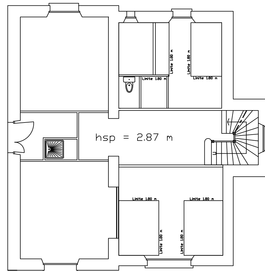
Comble
