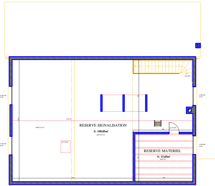
BATIMENT A PLAN DU 1er ETAGE
