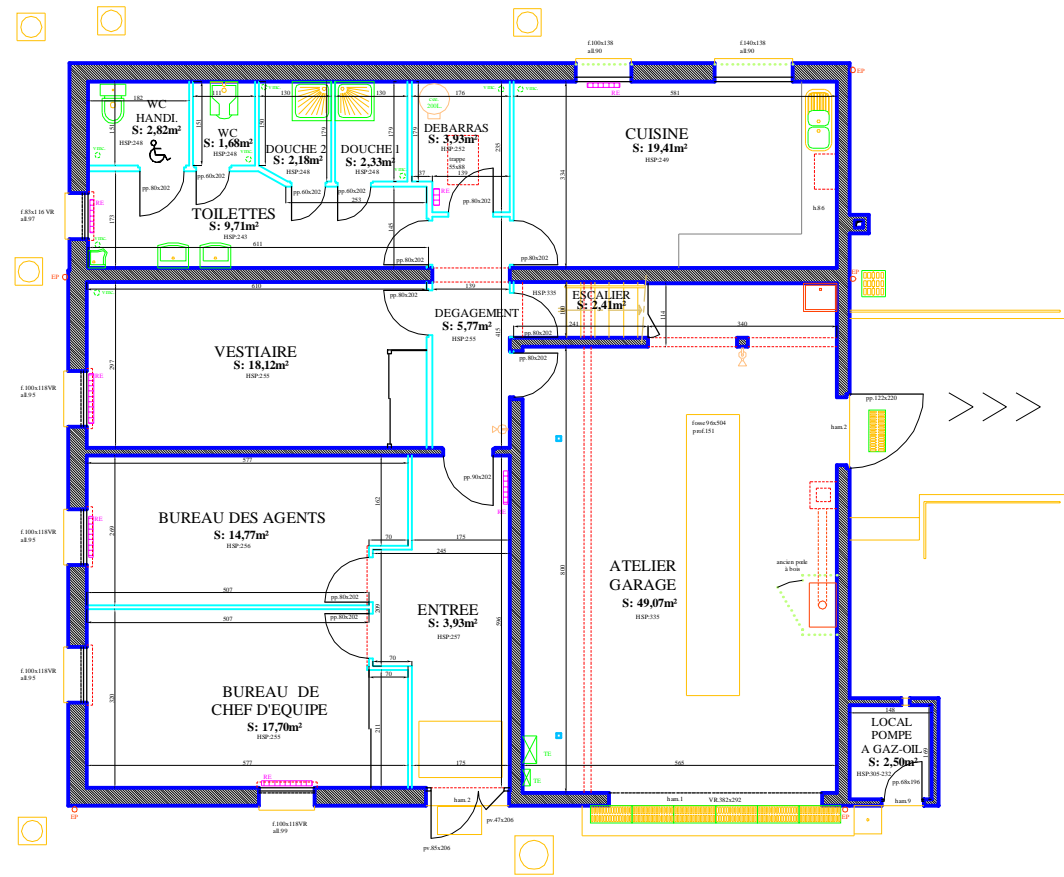
BATIMENT A PLAN DU REZ - DE - CHAUSSEE
