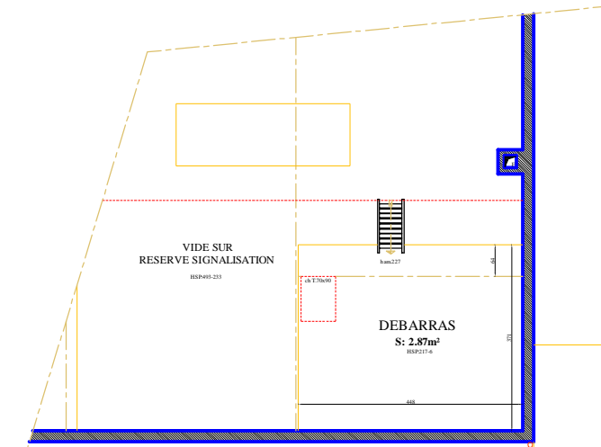
BATIMENT A PLAN DU 2e ETAGE
