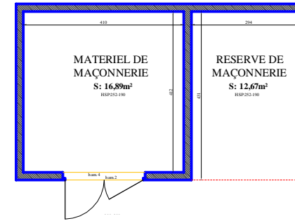
BATIMENT B PLAN DU REZ - DE - CHAUSSEE
